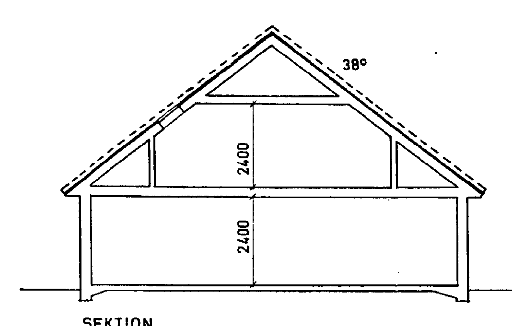
SEKTION
